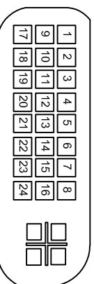
J17 (DVI-D)
